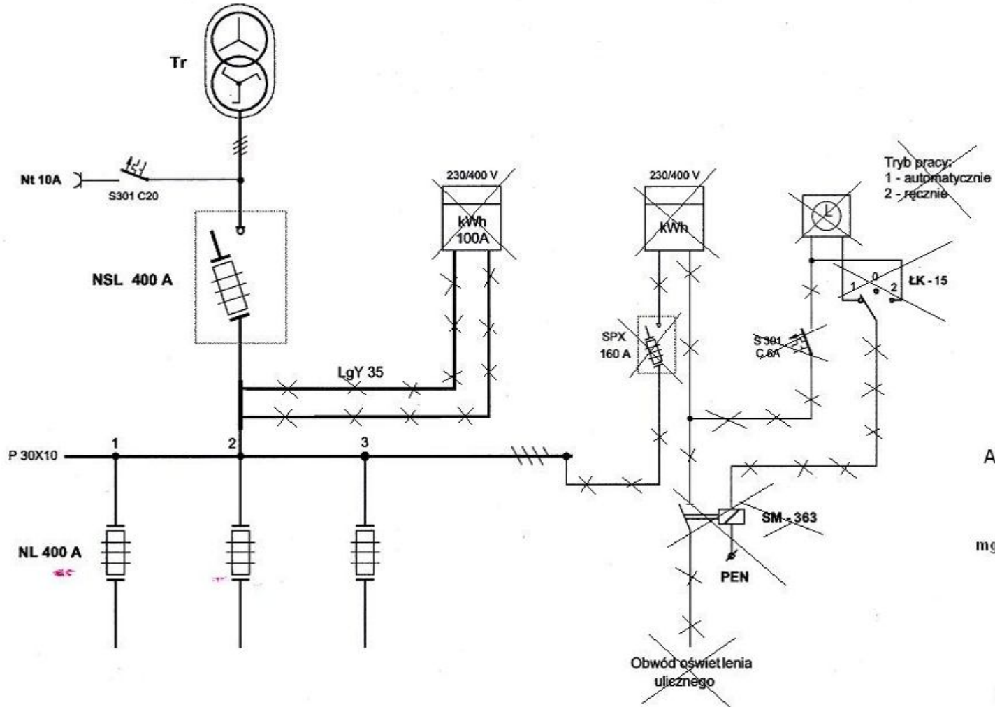
Schemat elektryczny rozdzielni RS 3 O/Pb
